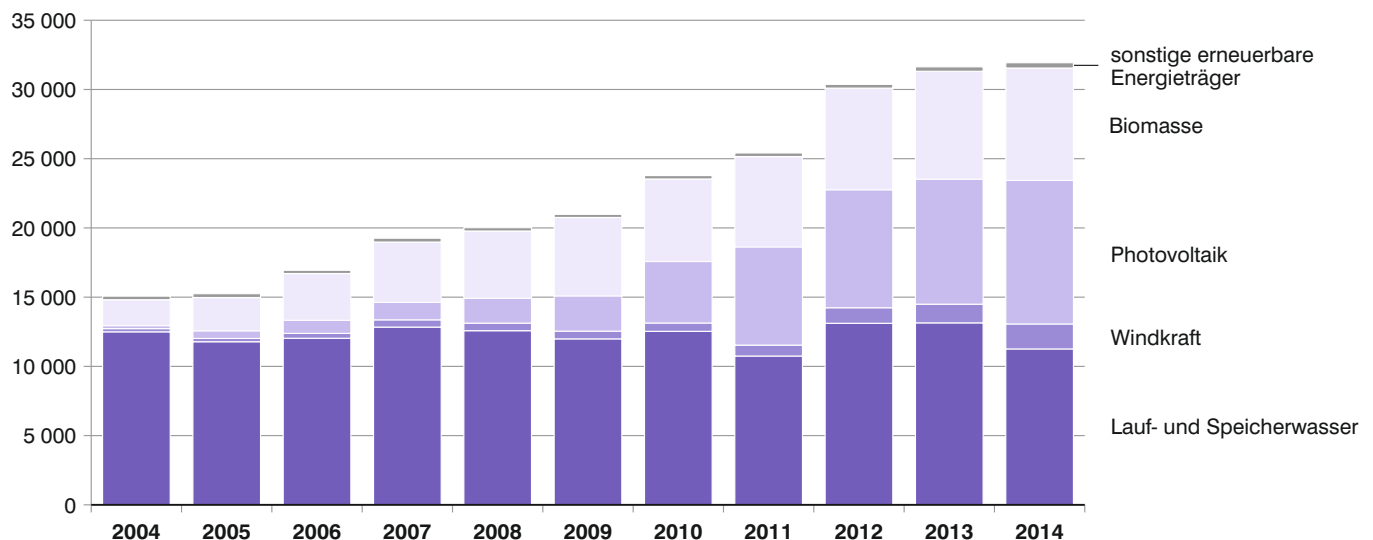
Abb. 12 Elektrizitätserzeugung aus erneuerbaren Energien in Bayern 2004 bis 2014 in GWh
