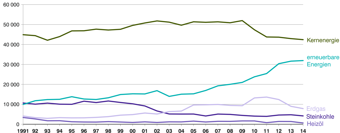
Abb. 5 Stromerzeugung in Bayern 1991 bis 2014 nach ausgewählten Energieträgern in Millionen kWh
