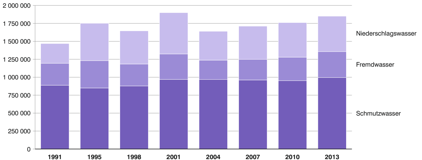
Abb. 9 Öffentliche Abwasserentsorgung in Bayern 1991 bis 2013 in 1 000 m 3
