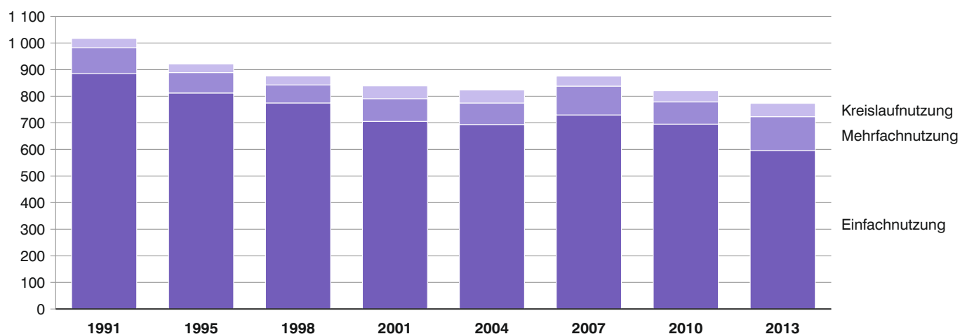
Abb. 8 Wasserverwendung des Bergbaus und der Gewinnung von Steinen und Erden sowie des Verarbeitenden Gewerbes in Bayern 1991 bis 2013 in 1 000 m 3
