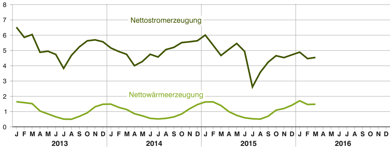
Strom- und Wärmeerzeugung (netto) in den Jahren 2013 bis 2016 in Millionen Megawattstunden (MWh)
