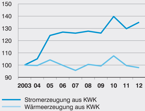
Strom- und Wärmeerzeugung* aus Kraft-Wärme-Kopplung** (KWK) 2003 \pm 100
